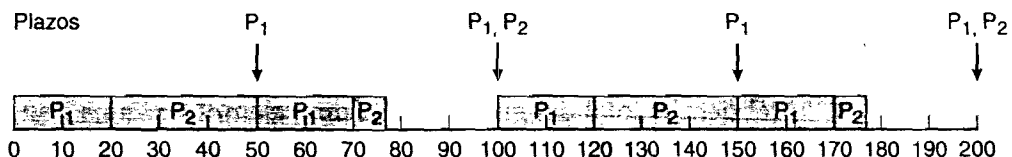
Figura 19.8 Planificación por prioridad monótona en tasa.
