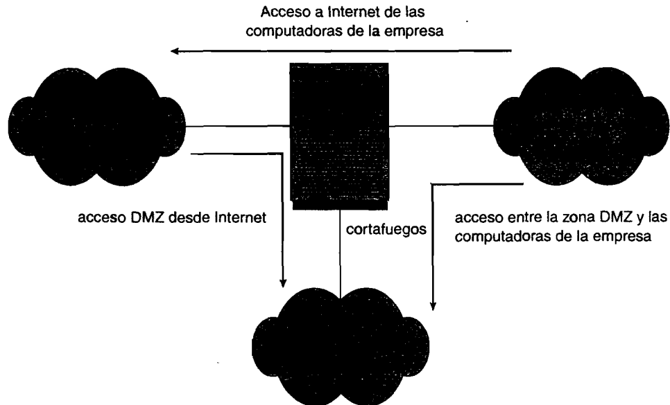
Figura 15.10 Separación de dominios mediante un cortafuegos.
