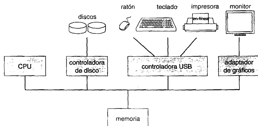
Figura 1.2 Una computadora moderna.
