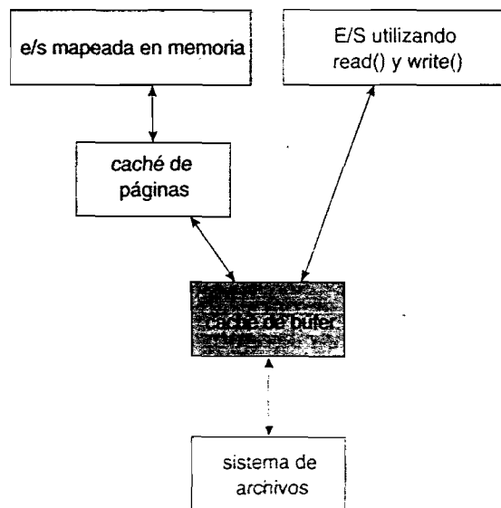
Figura 11.11 E/S sin una caché de búfer unificada.
