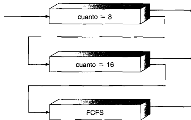
Figura 5.7 Colas multinivel realimentadas.
