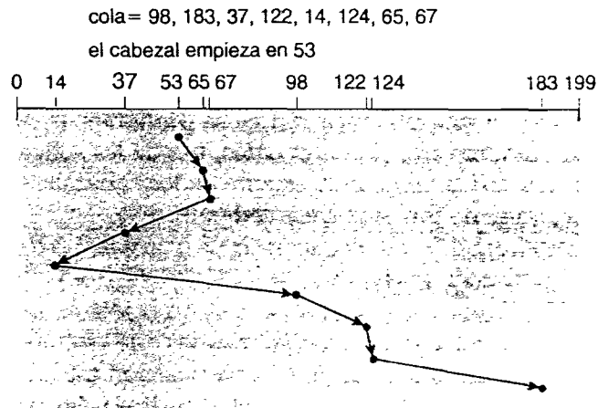
Figura 12.5 Planificación SSTF de disco.
