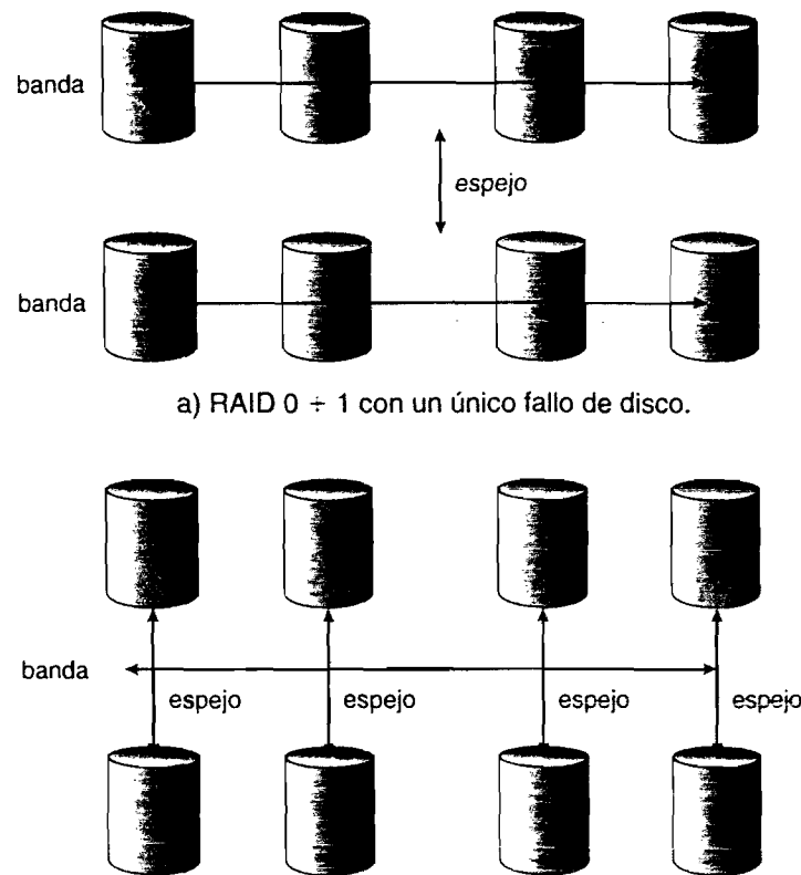
b) RAID 1 + 0 con un único fallo de disco.
