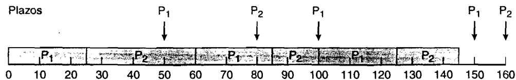
Figura 19.10 Planificación por prioridad en finalización de plazo.
