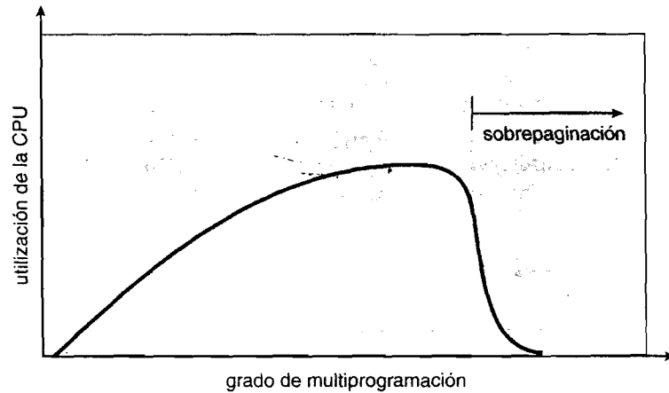
Figura 9.18 Sobrepaginación.
