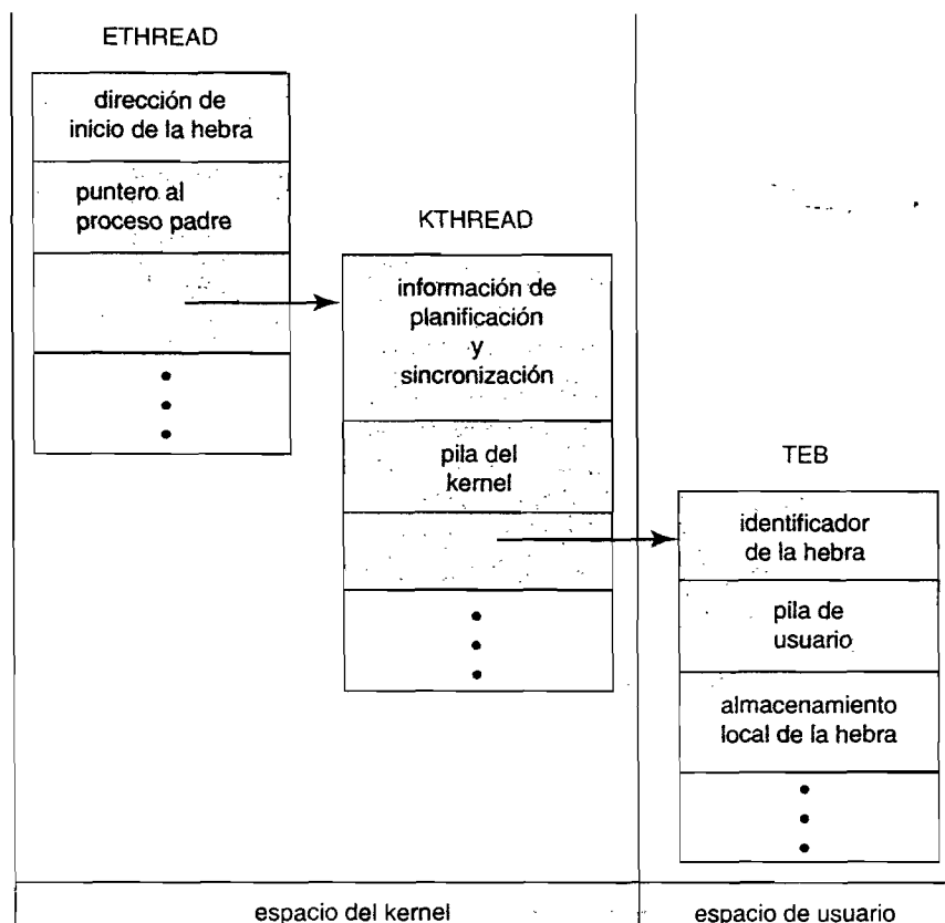
Figura 4.10 Estructuras de datos de una hebra de Windows XP.
