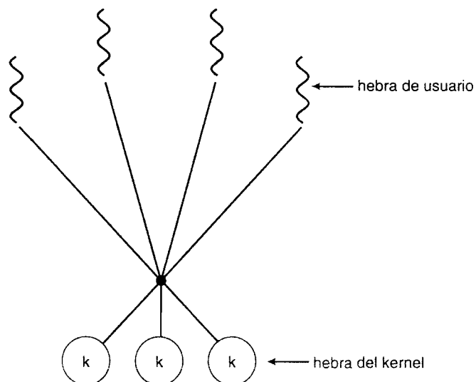
Figura 4.4 Modelo muchos-a-muchos.
