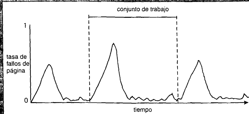
Figura 9.22. Tasa de fallos de página en función del tiempo.
