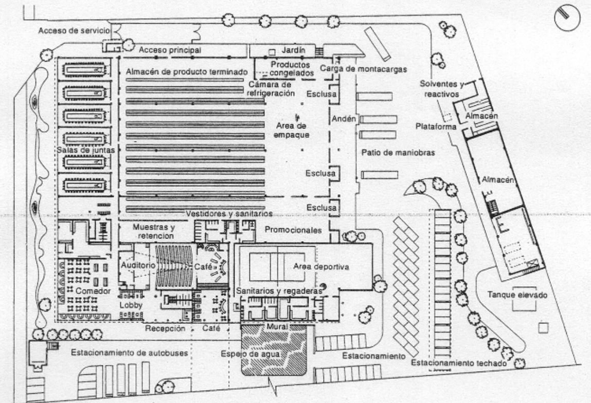
Planta general almacén
