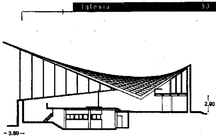
Corte longitudinal
