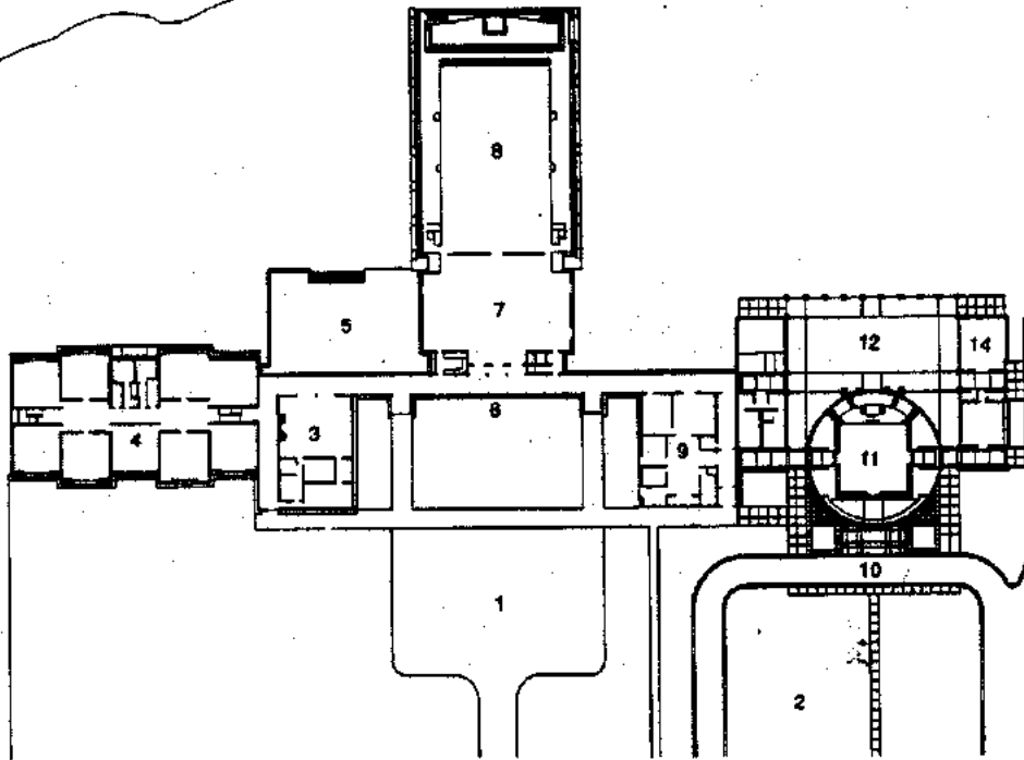
Planta general
