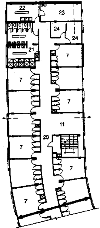
Planta alta cuerpo B
