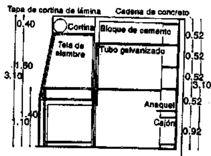
Corte
