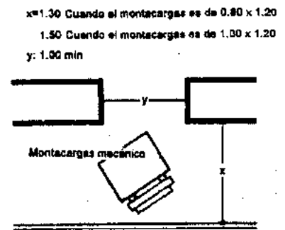
Maniobras en pasillo y dimensiones de montacarga
