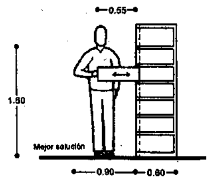
Arrastre de cajones de almacenamiento
