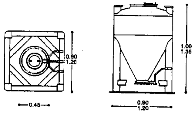
Recipiente fármaco, para granulados
