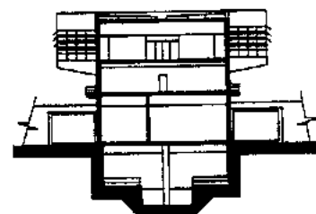
Corte torre de observación
