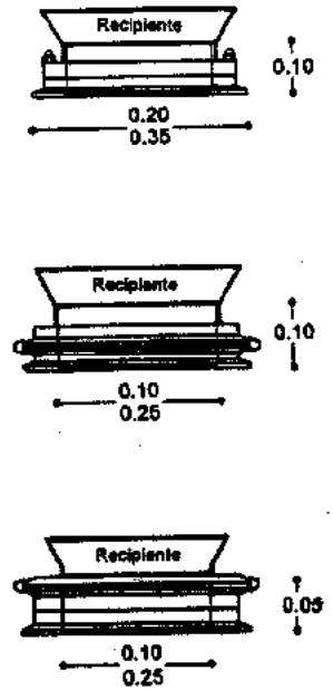
Válvulas mariposas para recipientes fármacos
