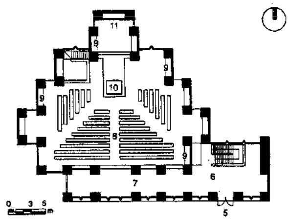
Planta principal
