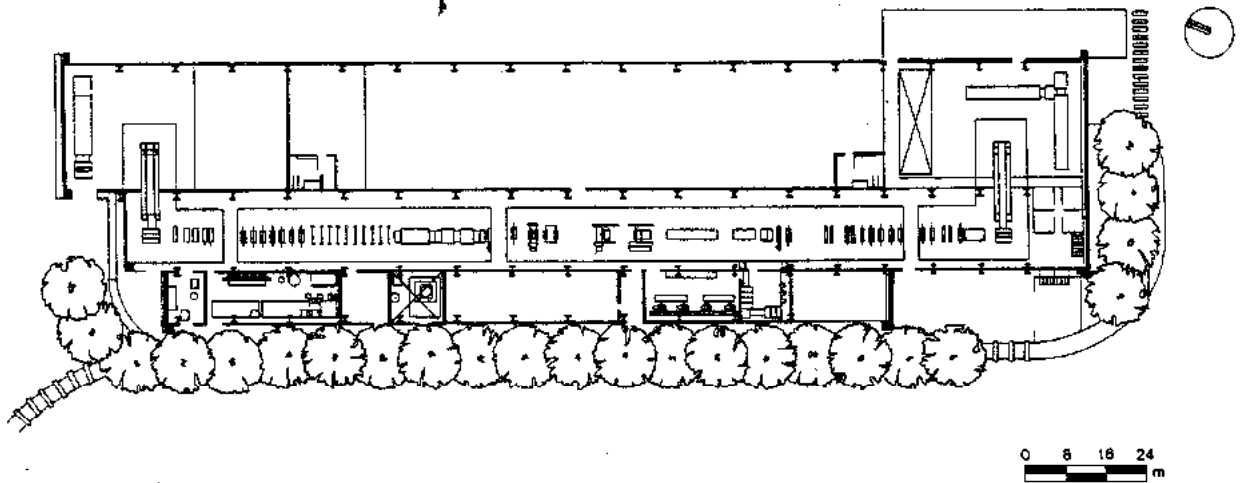
Planta general
