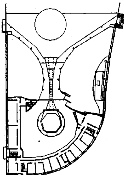
Planta alta
