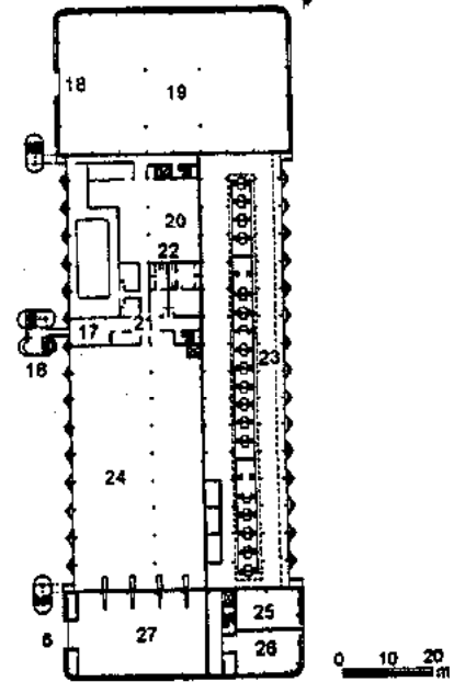
Planta baja general
