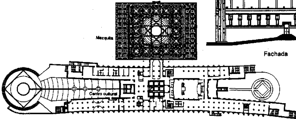
Planta general
