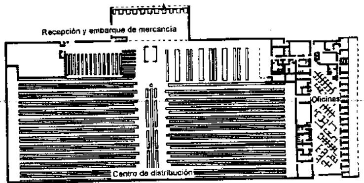
Planta general
