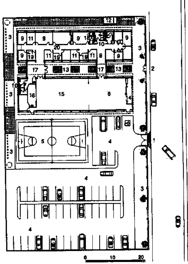
Planta baja solución A (ampliación)
