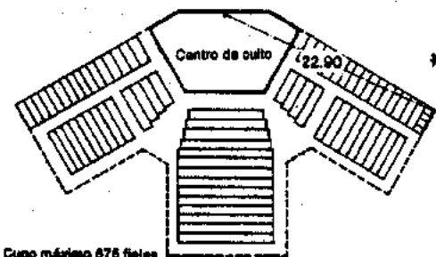
Solución de asientos tipo auditorio, nave de tres aias
