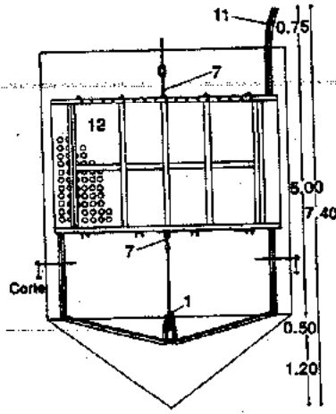
Alzado
