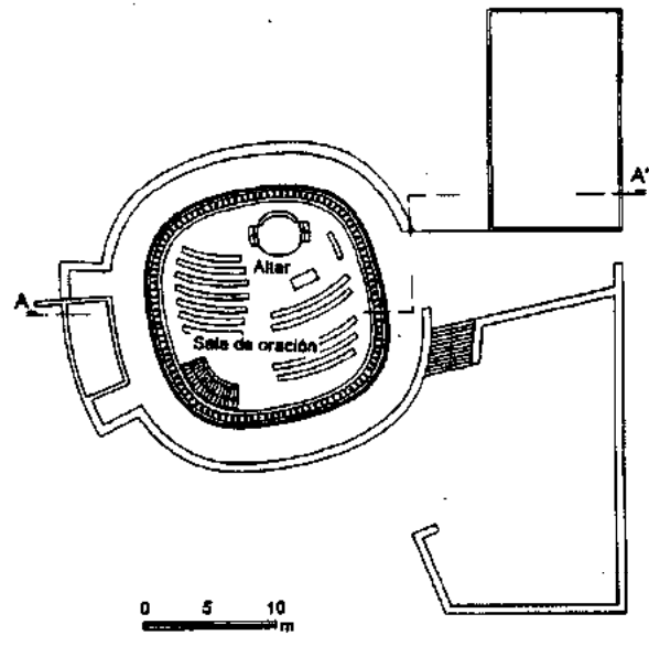
Planta alta
