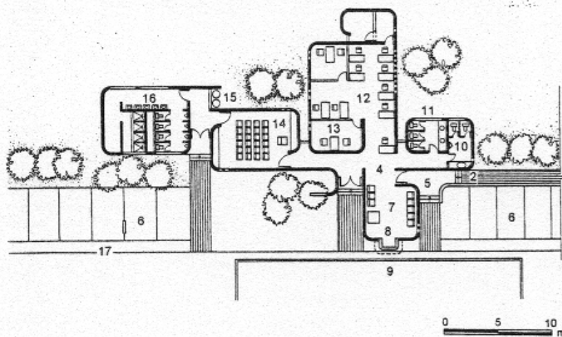
Planta edificio de oficinas
