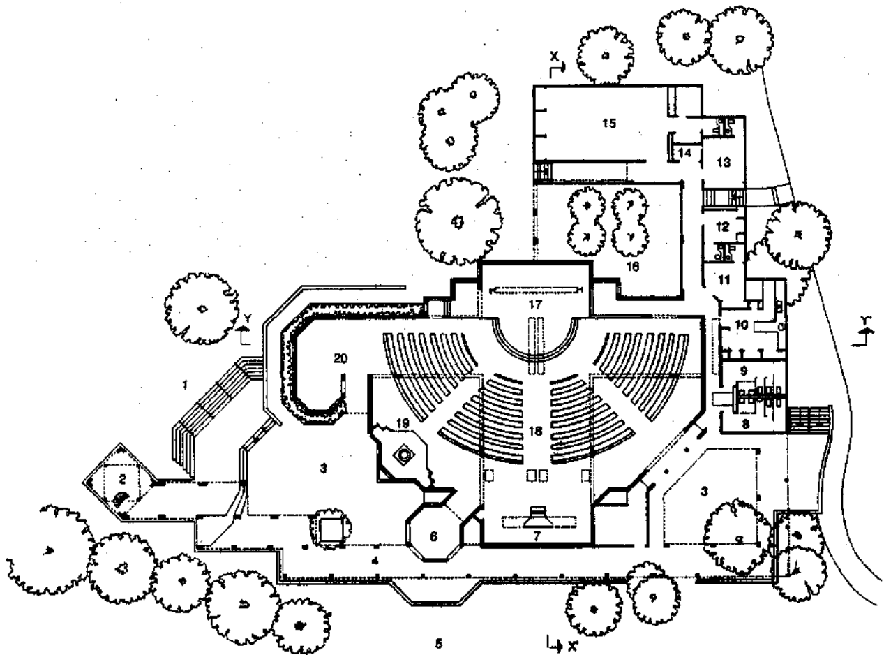
Planta general
