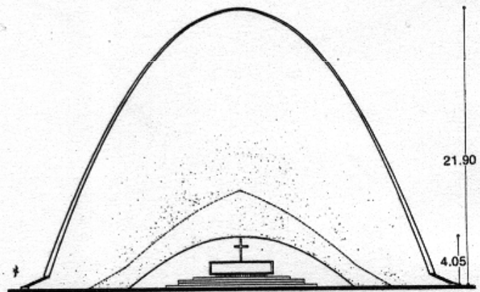
Fachada frontal
