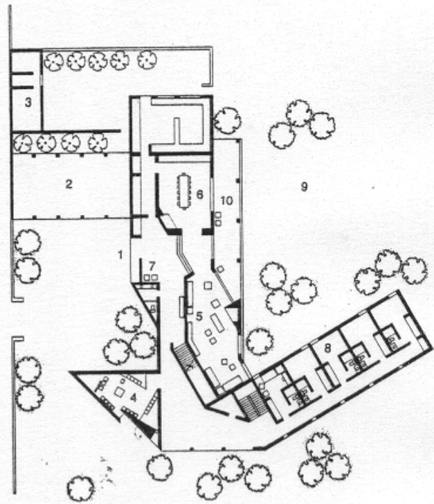
Planta general
