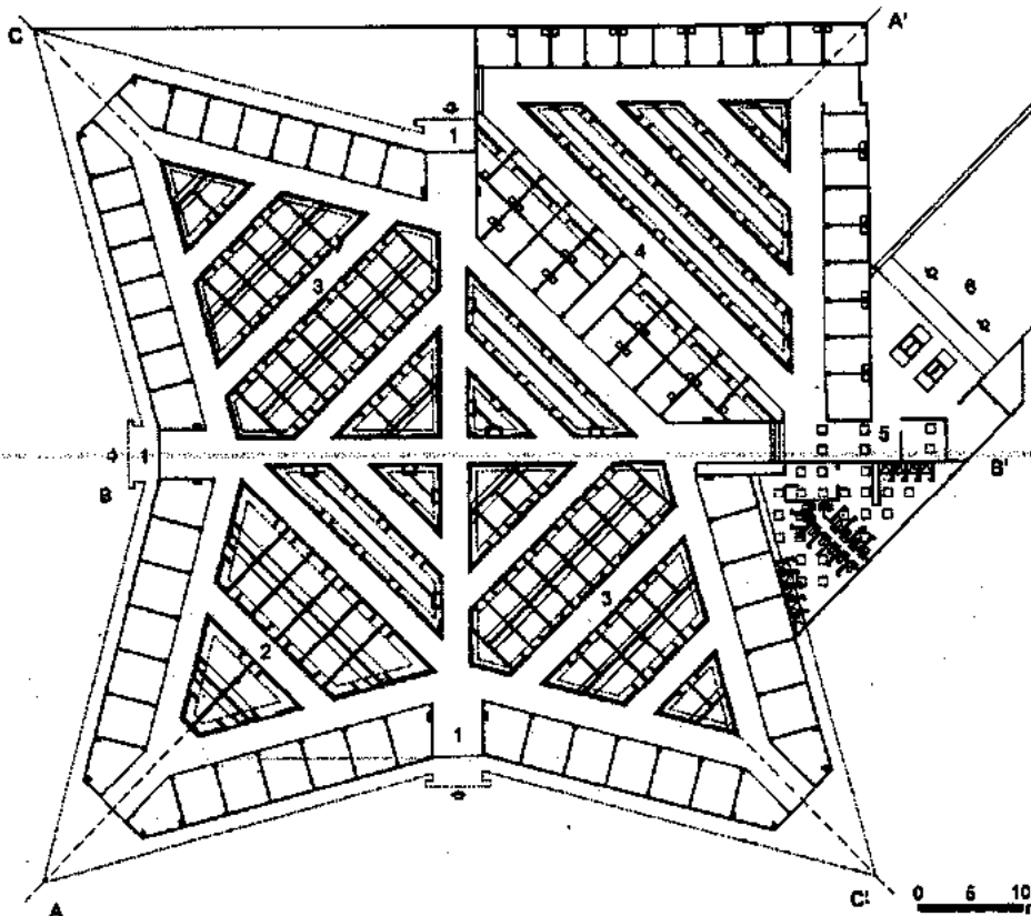
Planta general
