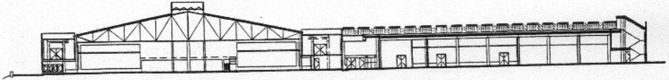
Corte transversal
