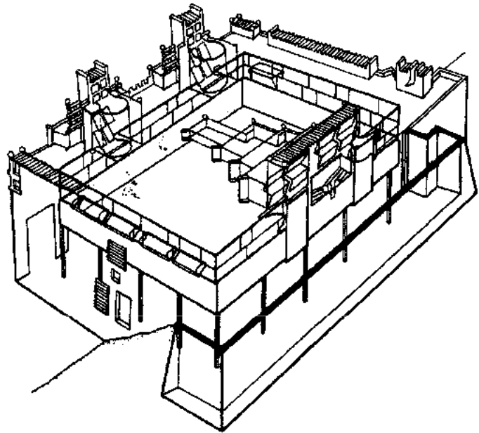
Isométrico área procesadora
