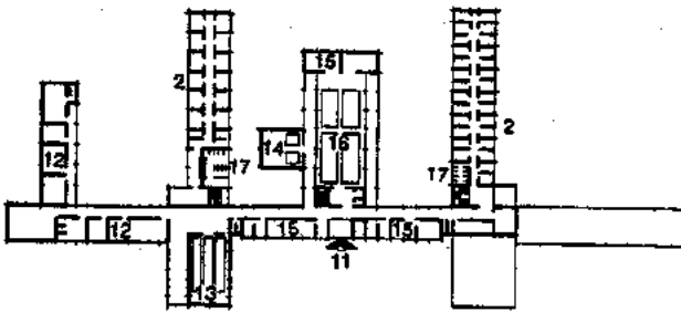
Planta baja
