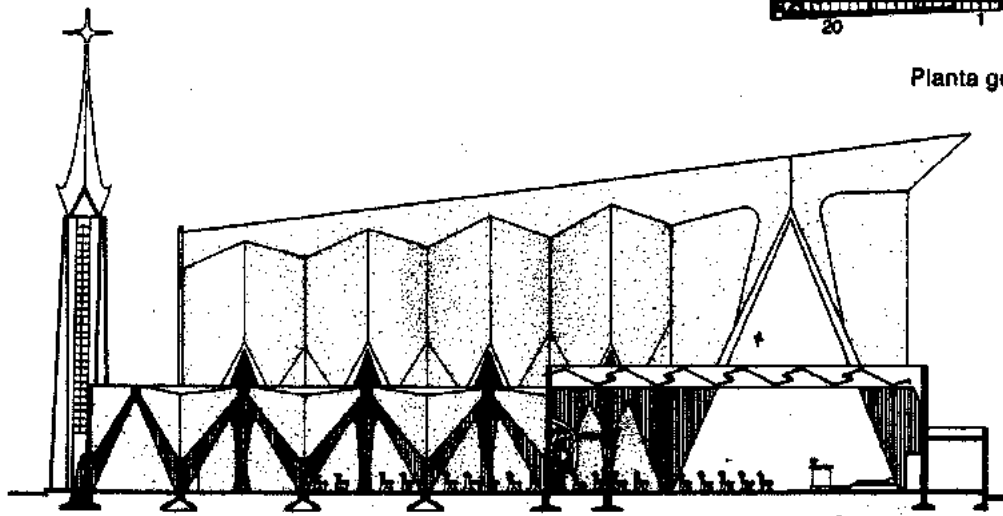
Corte longitudinal
