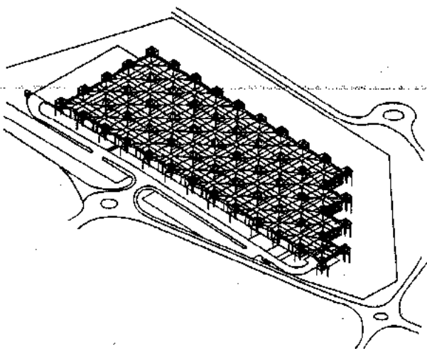
Perspectiva conjunto
