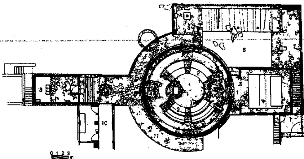
Planta general
