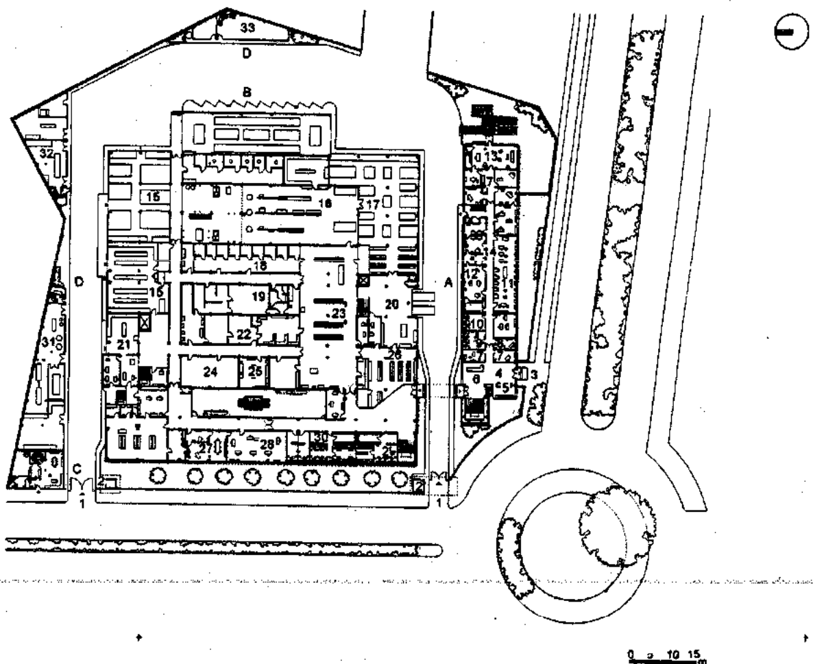
Planta de acceso
