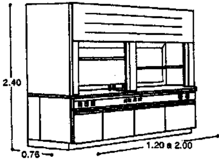
Campana de humos para ácido perclórico
