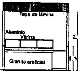
Alzado
