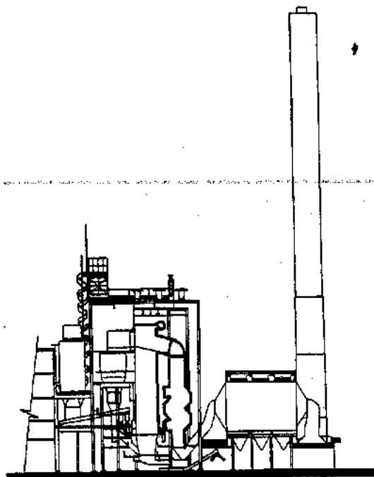
Corte
