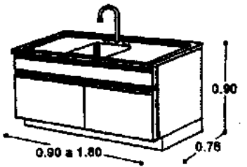
Fregadero de cabecera con cubierto y tarja sin accesorios
