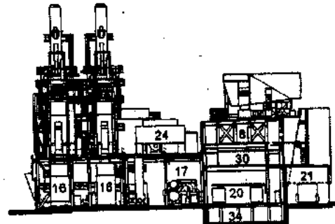
Corte C-C'
