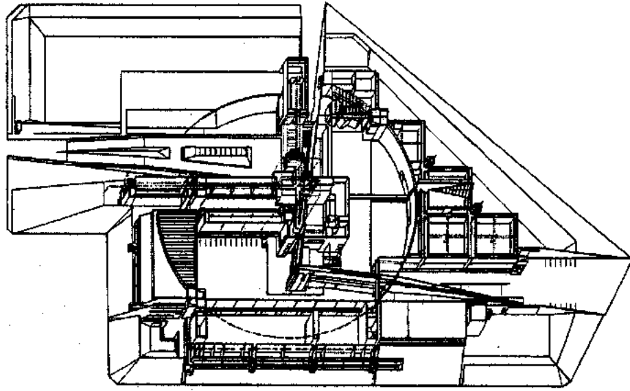
Axonométrico
