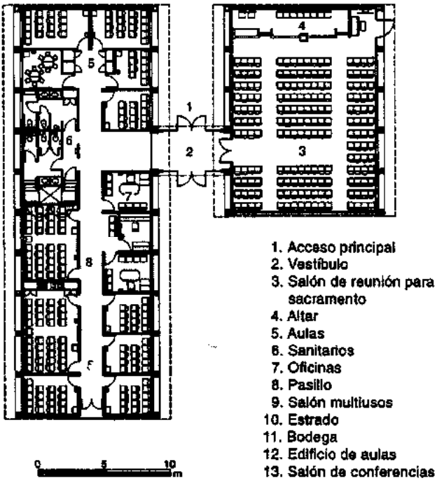
Planta baja (primera etapa)
