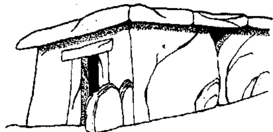
Megalito
