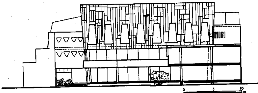
Fachada posterior
