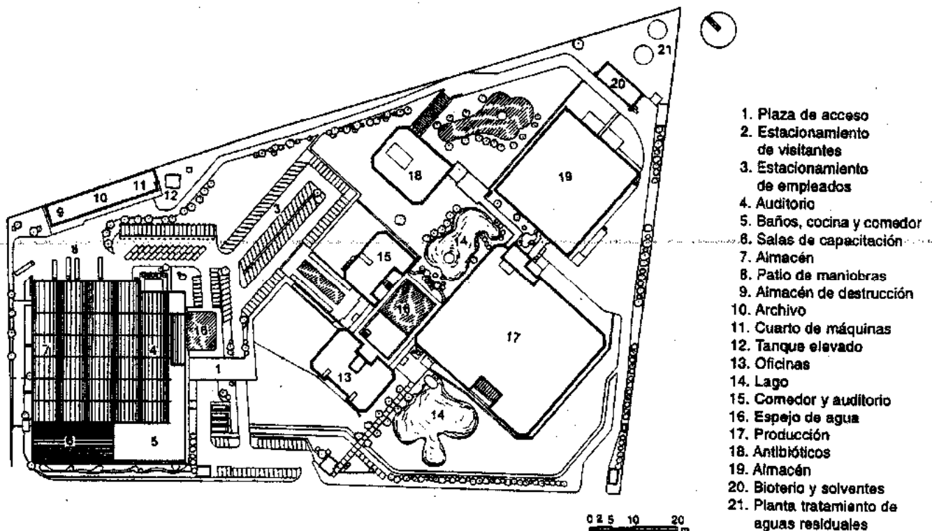
Planta general
