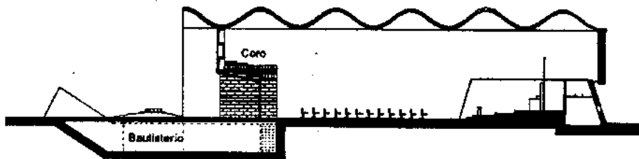
Corte longitudinal
