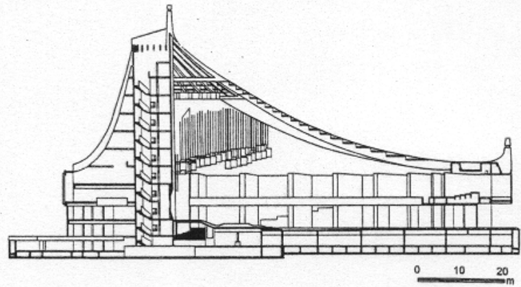
Corte
