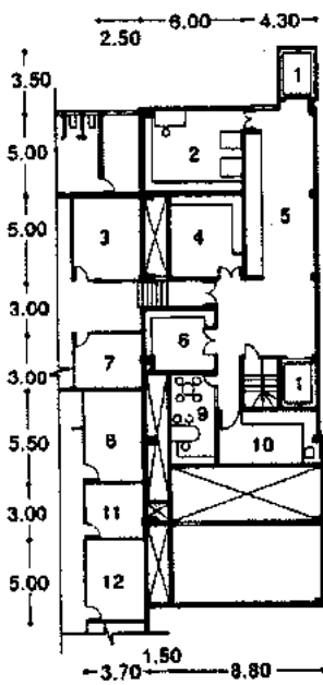
Planta servicios
