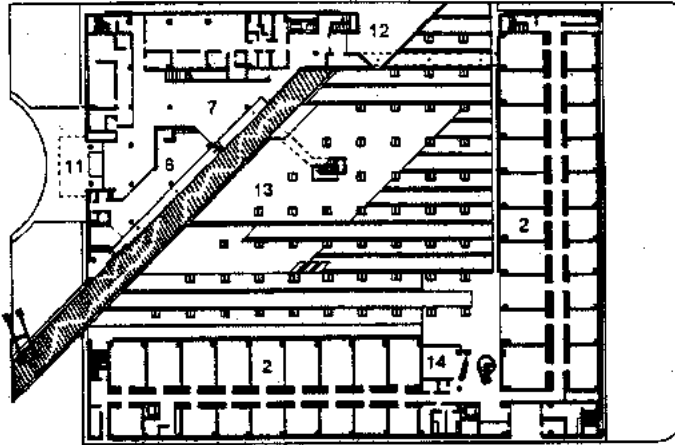
Planta baja
