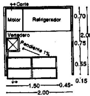
Planta
