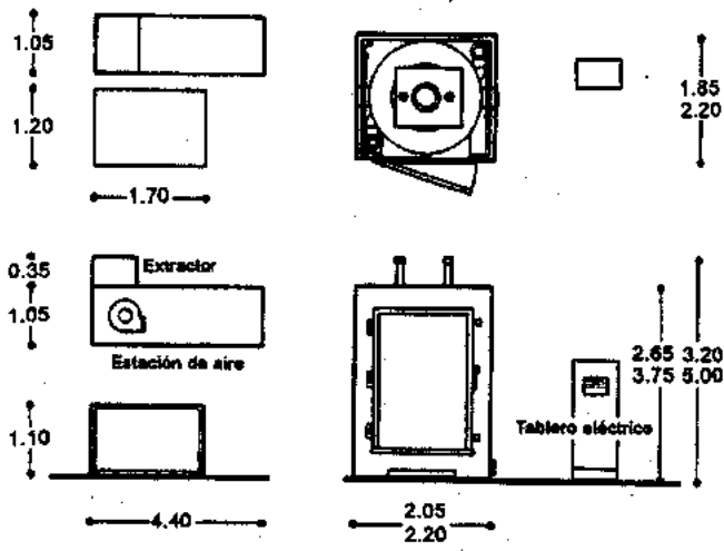
Estación de lavado y secado de utensilios automático
