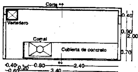
Planta
