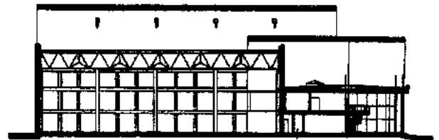
Corte longitudinal
