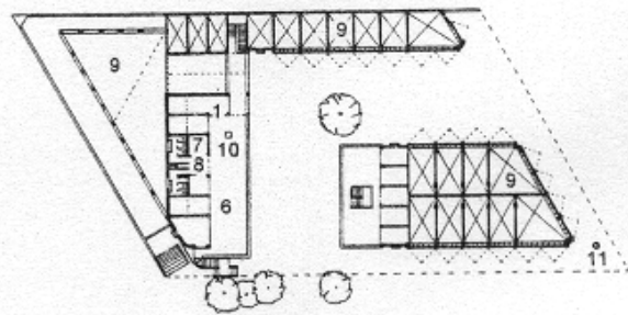
Planta alta
