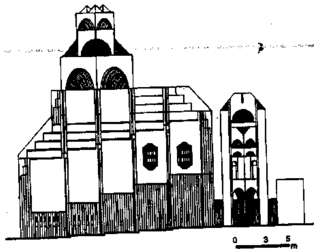
Fachada
