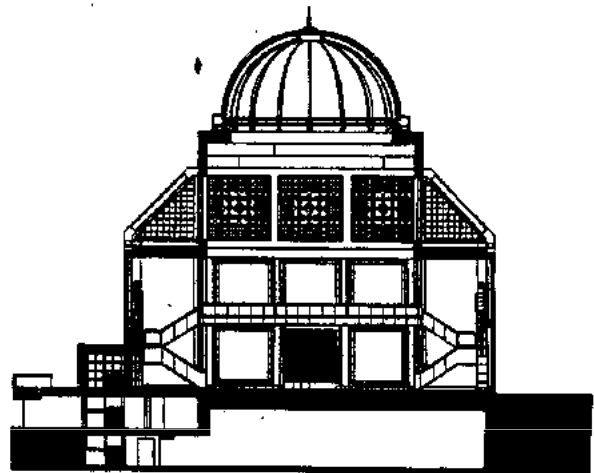
Corte
