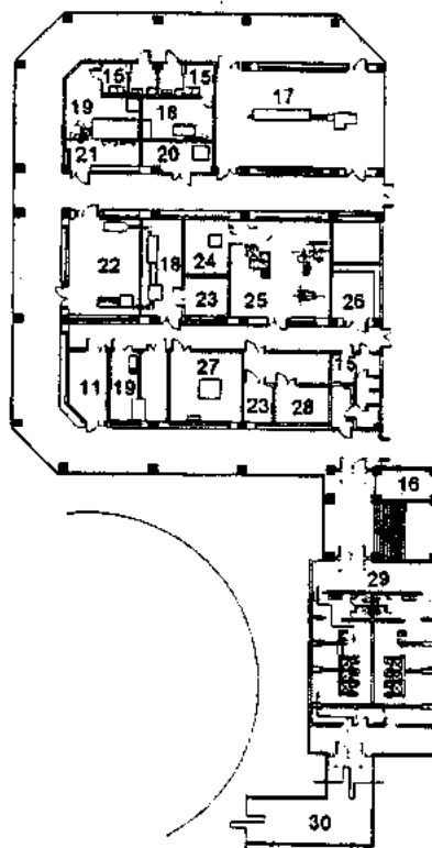
Planta baja (antibióticos)
