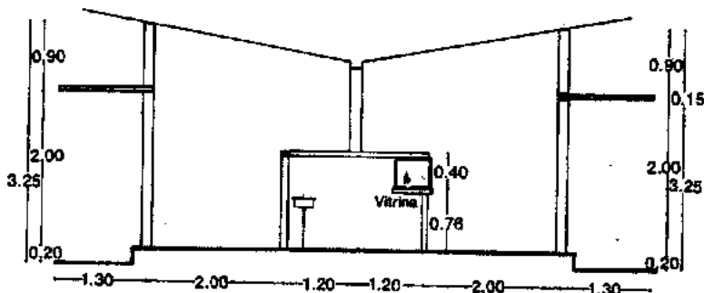
Alzado general
