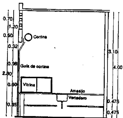
Corte
