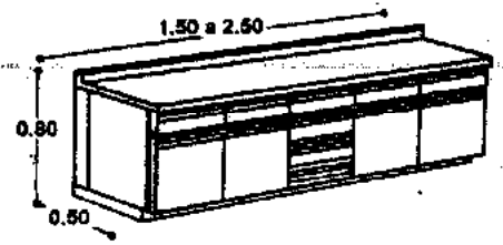
Fregadero de cabecera con cubierto y tarja sin accesorios
