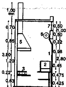
Corte
