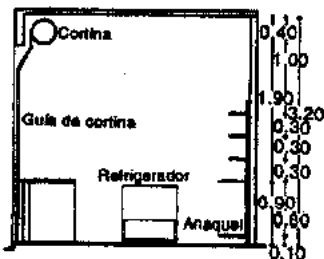
Corte
