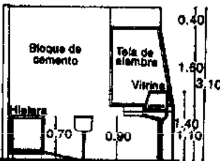
Corte
