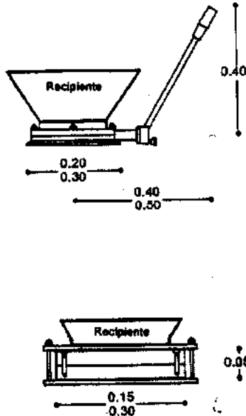
Válvulas mariposas para recipientes fármacos
