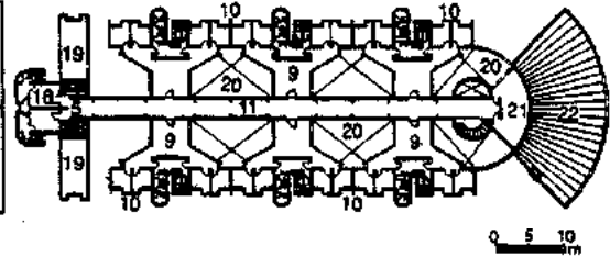
Planta alta edificio de residencia Filosofía
