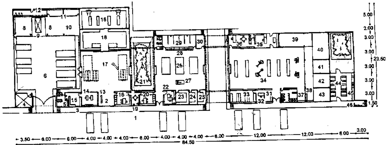
Planta baja
