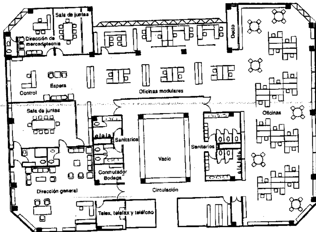
Planta alta oficinas
