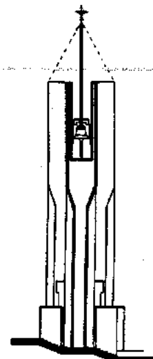
Plantas y corte del campanario
