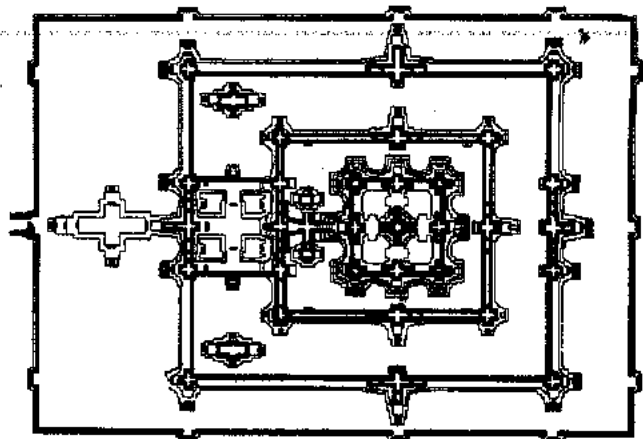
Planta general
