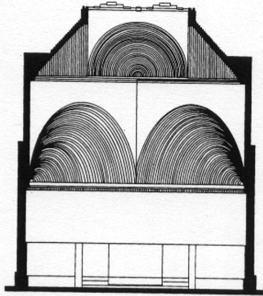
Corte
