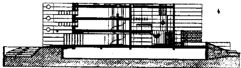
Corte longitudinal
