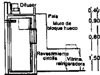
Alzado y corte Garnicería
