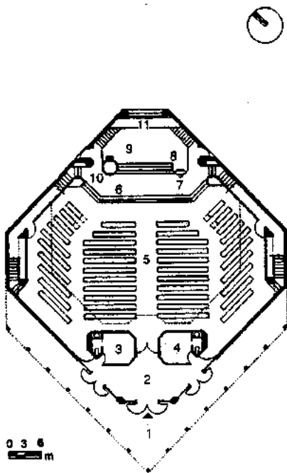
Planta general
