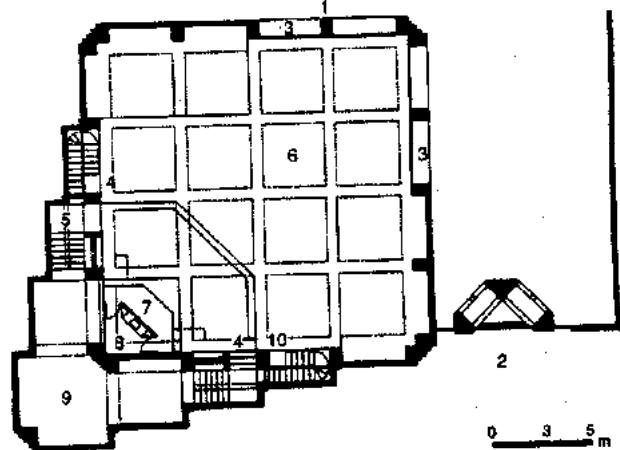
Planta principal
