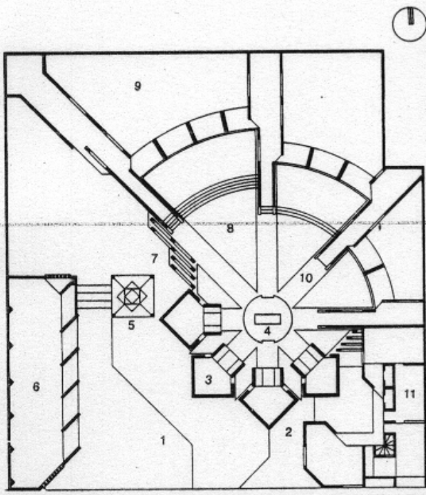
Planta general
