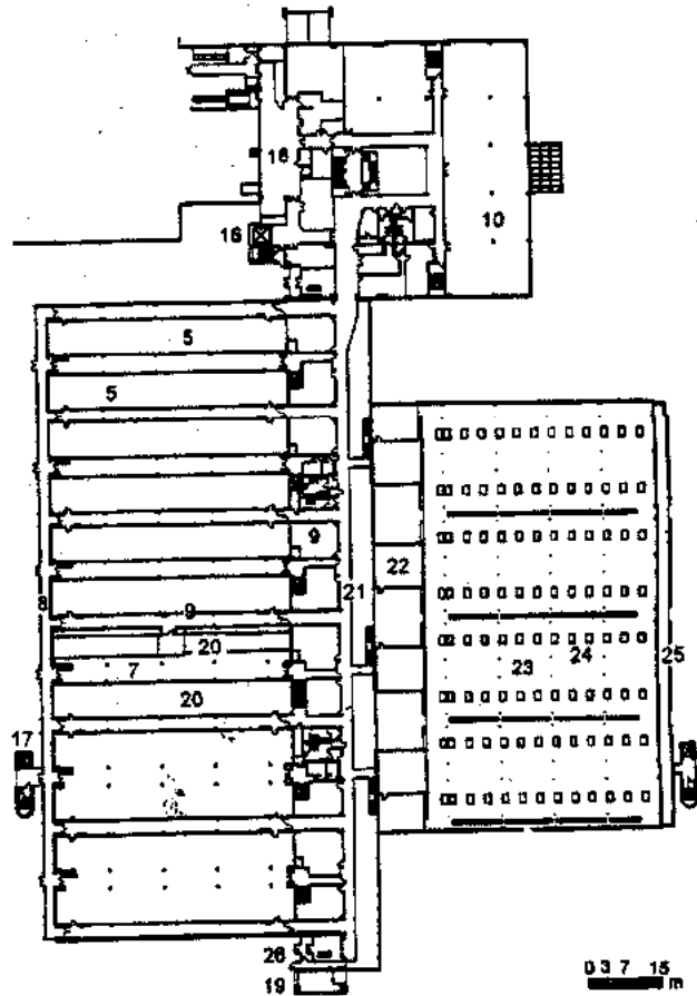
Planta segundo piso
