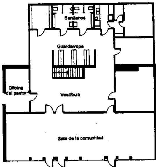
Planta sótano
