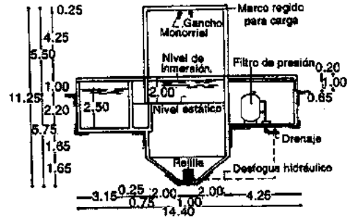
Corte 2
