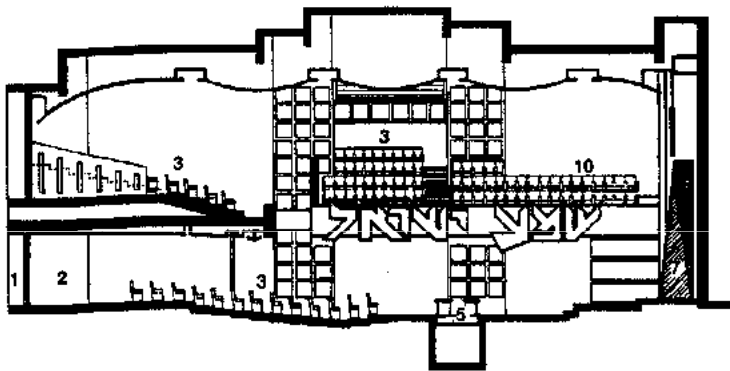
Corte longitudinal
