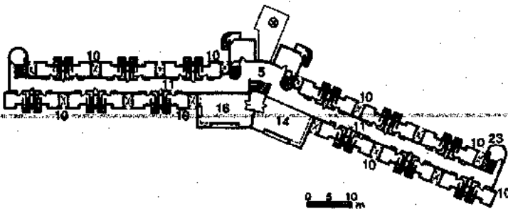
Planta alta edificio de residencia Teología
