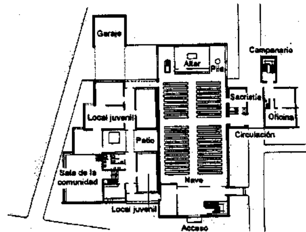
Planta general
