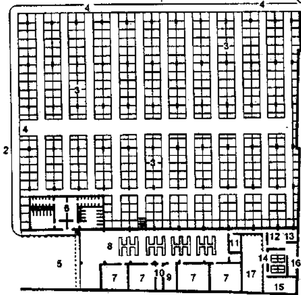
Planta general
