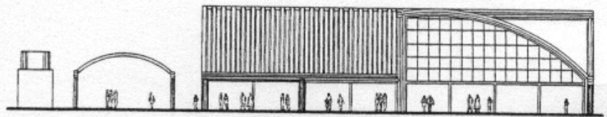
Fachada
