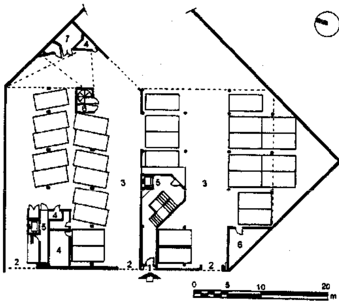
Planta baja
