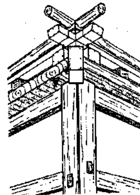
Detalle de la esquina del Santuario Izumo
