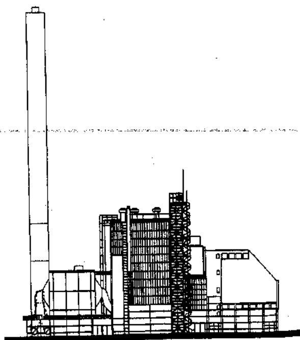
Fachada
