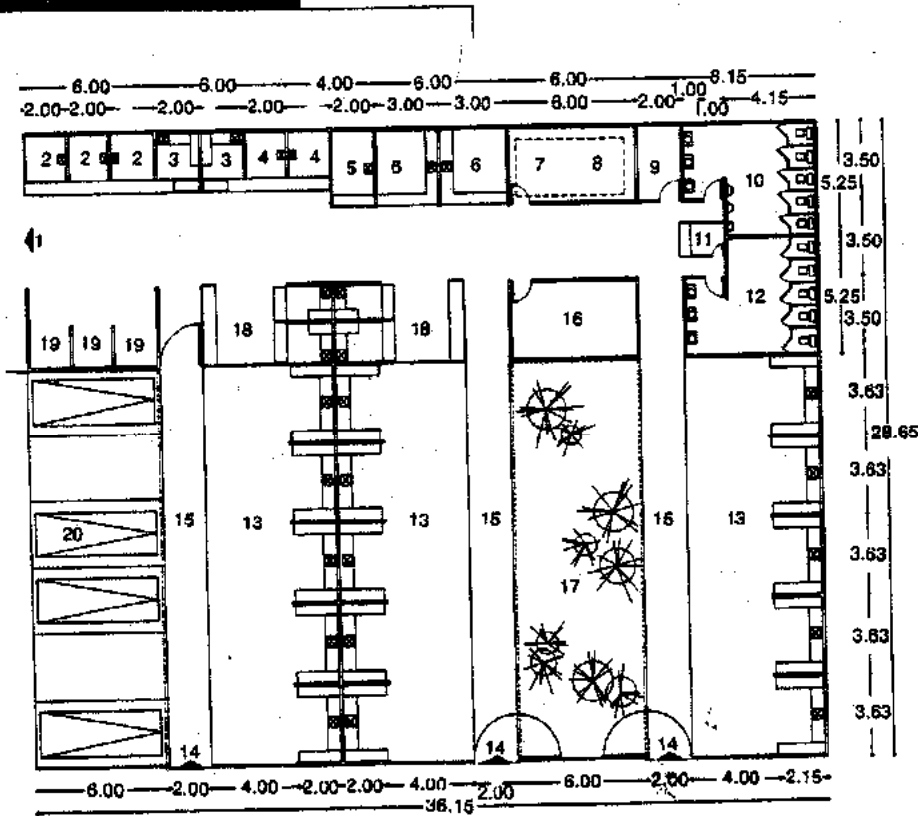
Planta
