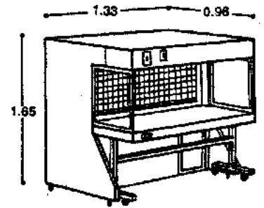
Campana de flujo laminar
