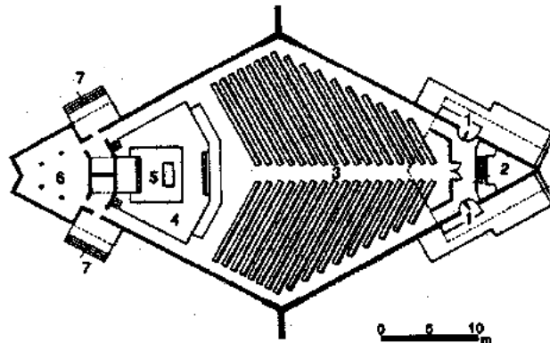
Planta general
