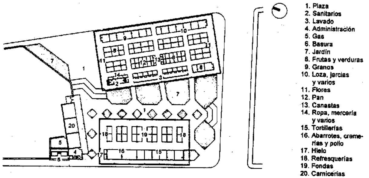
Planta general
