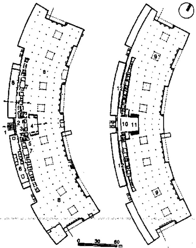
Planta baja
