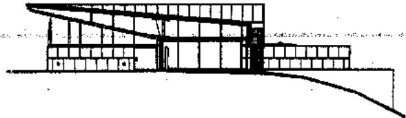
Fachada suroeste
