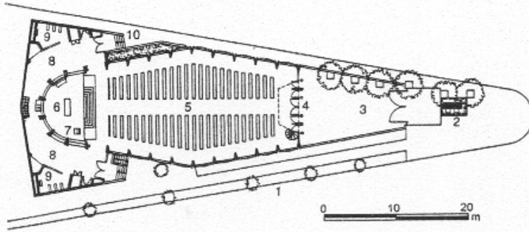
Planta general
