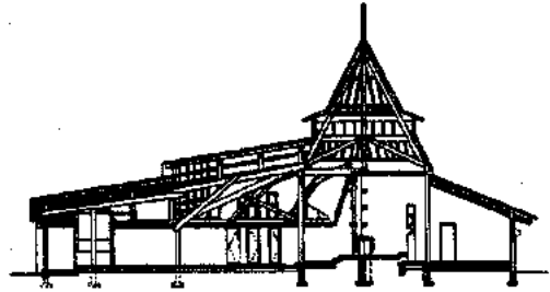
Corte
