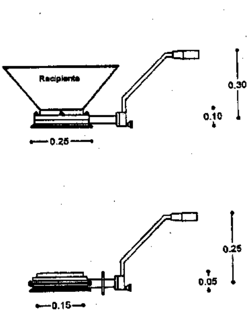
Válvulas con recipiente para tabletas
