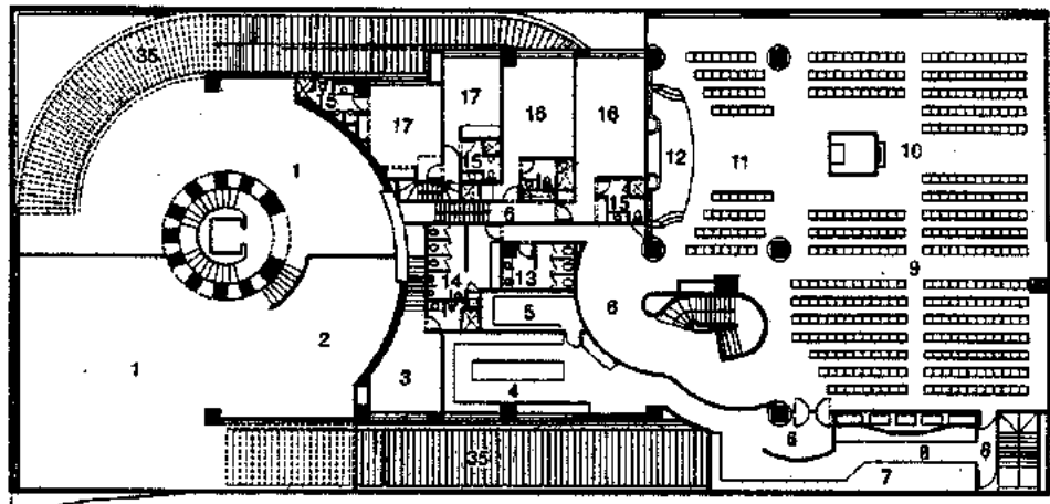
Planta semisótano
