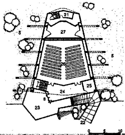
Planta principal. Capilla auditorio
