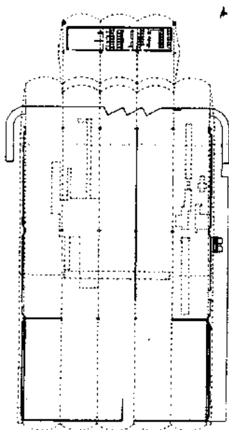
Planta general
