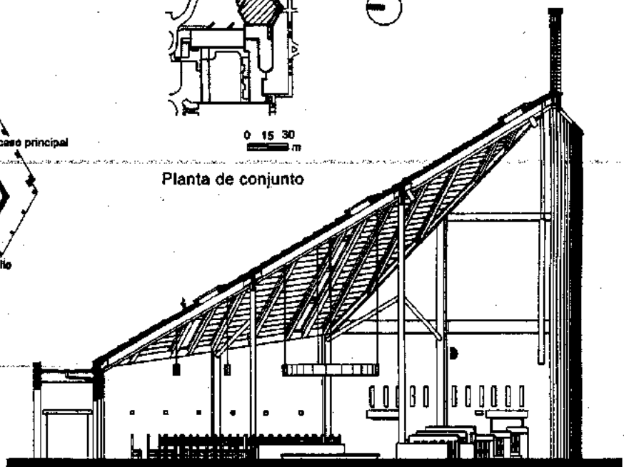
Corte
