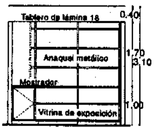
Alzado
