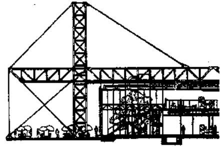
Detalle corte
