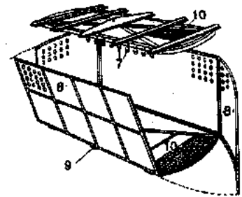
Isométrico
