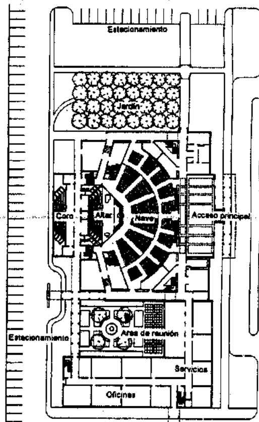
Planta principal
