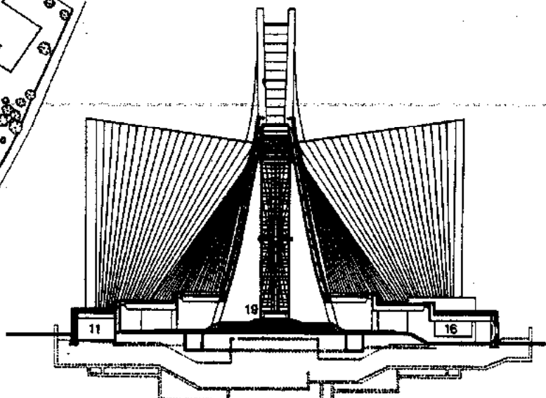
Corte transversal
