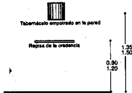
Alzado de sagrario y credencia
