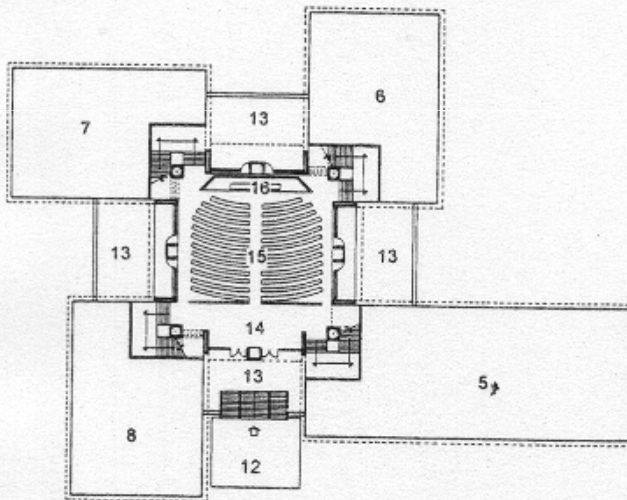
Planta nivel basamento
