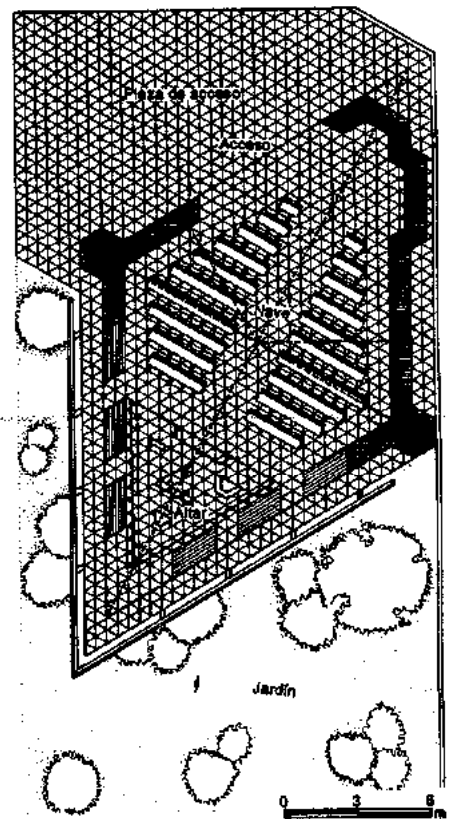
Planta baja
