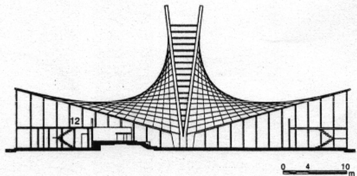
Corte longitudinal
