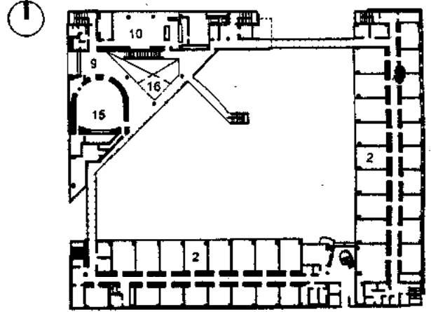
Planta alta
