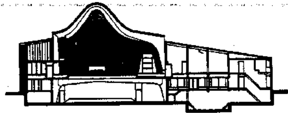
Corte longitudinal
