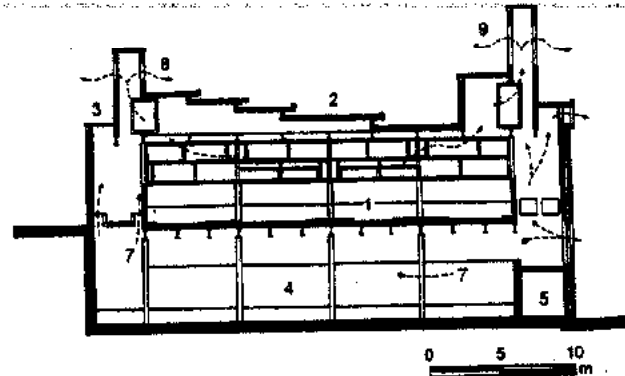
Corte ventilación de noche
