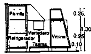
Corte
