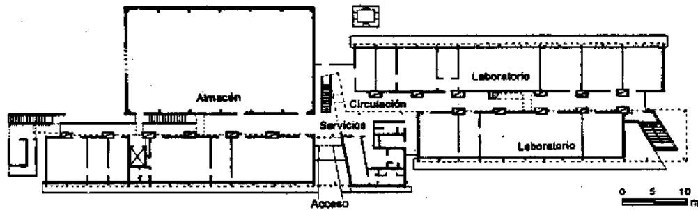
Planta general
