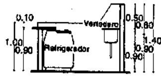
Corte
