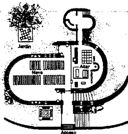
Planta general
