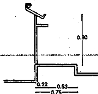
Planta y alzado de bancas con reclinatorio
