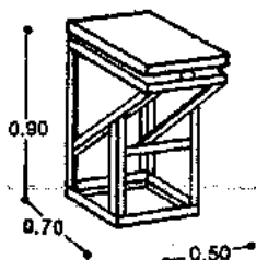
Emplazamiento para balanza analítica
