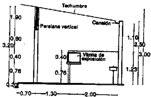
Corte
