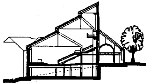
Corte
