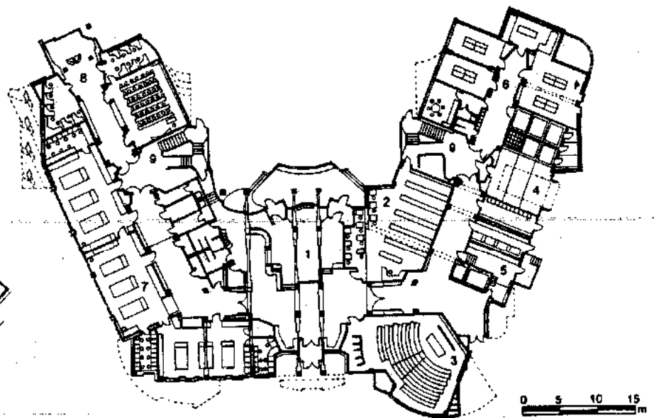
Planta general
