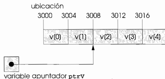
Figura 7.19 El apuntador ptrV después de aplicar la aritmética de apuntadores.
