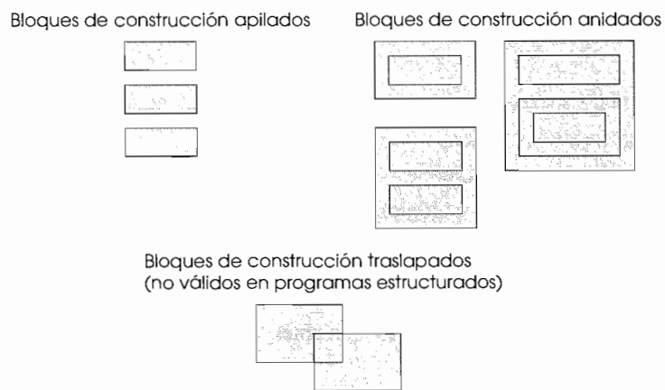
Figura 4.22 Bloques de construcción apilados, anidados y traslapados.
