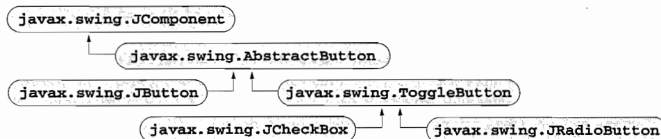
Figura 29.10 La jerarquía de botones.
