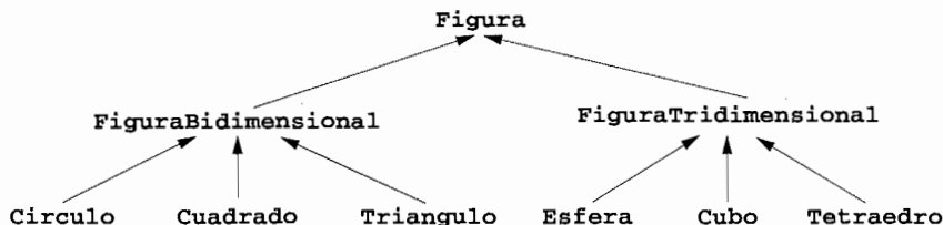
Figura 27.2 Una parte de la jerarquía de la clase Figura .
