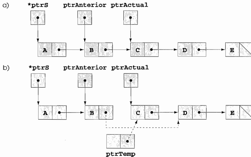
Figura 12.6 Eliminación de un nodo de una lista.
