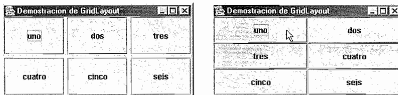
Figura 29.19 Programa que muestra el uso de componentes en GridLayout ; DemoGridLayout.java . (Parte 2 de 2.)
