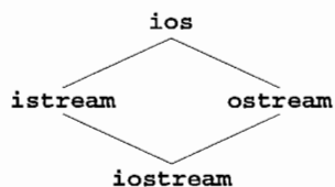
Figura 21.1 Parte de la jerarquía de la clase de E/S de flujo.
