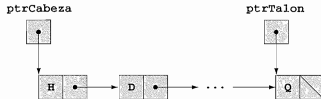
Figura 12.12 Representación gráfica de una cola.
