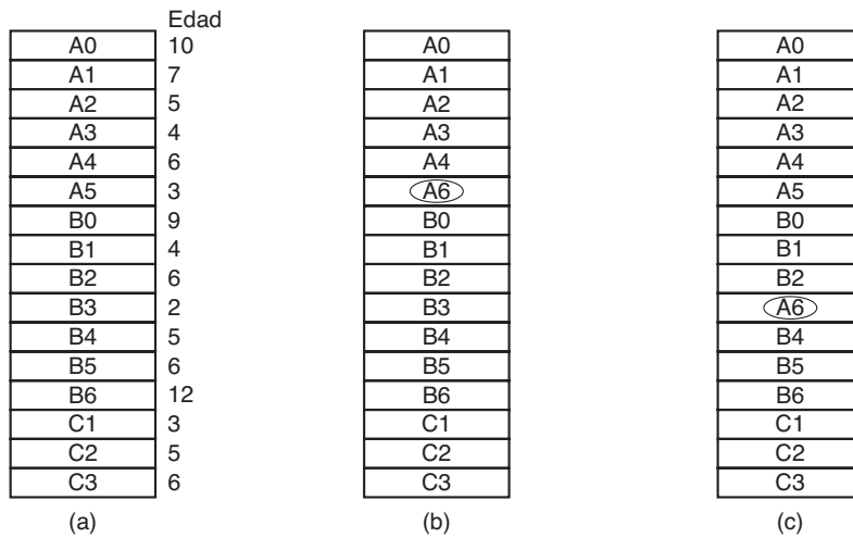
Figura 3-23. Comparación entre el reemplazo de páginas local y el global. (a) Configuración original. (b) Reemplazo de páginas local. (c) Reemplazo de páginas global.
