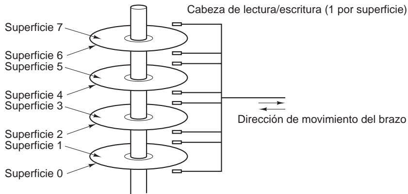
Figura 1-10. Estructura de una unidad de disco.
