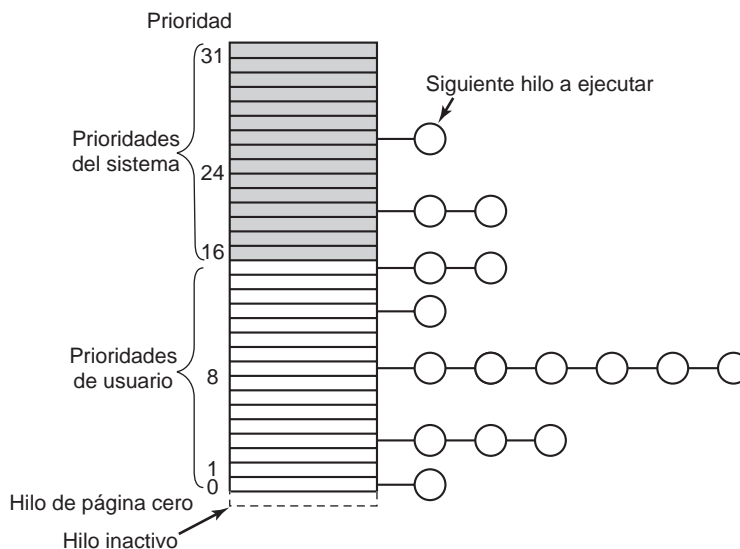
Figura 11-28. Windows Vista proporciona 32 prioridades para los hilos.
