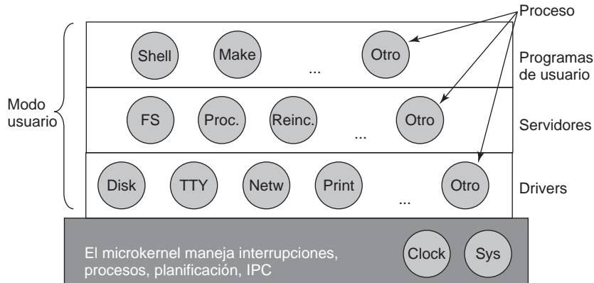
Figura 1-26. Estructura del sistema MINIX 3.
