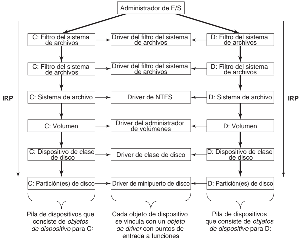
Figura 11-16. Representación simplificada de las pilas de dispositivos para dos volúmenes de archivos NTFS. EL paquete de peticiones de E/S se pasa desde la parte inferior de la pila. Se hacen llamadas a las rutinas apropiadas de los drivers asociados en cada nivel de la pila. Las mismas pilas de dispositivos consisten en objetos de dispositivo que se asignan de manera específica a cada pila.
