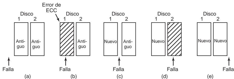
Figura 5-31. Análisis de la influencia de fallas en escrituras estables.
