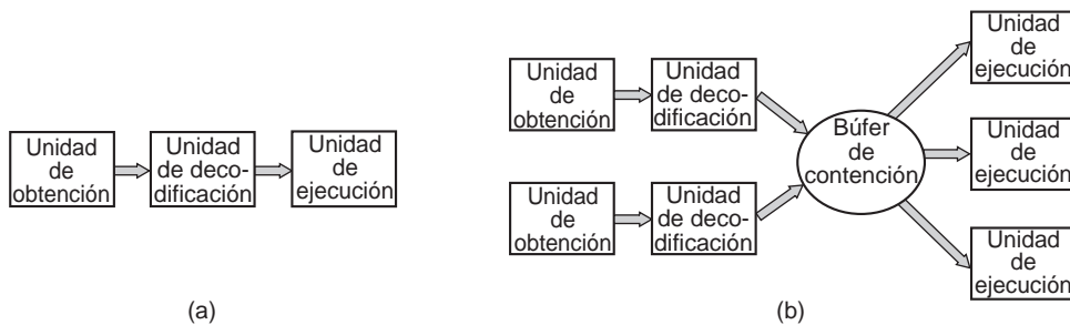
Figura 1-7. (a) Canalización de tres etapas; (b) CPU superescalador.
