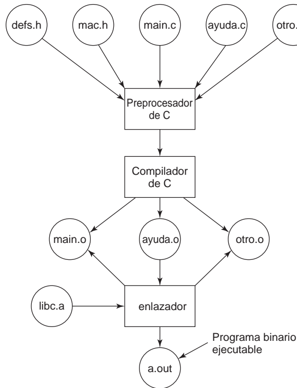
Figura 1-30. El proceso de compilar archivos de C y de encabezado para crear un archivo ejecutable.
