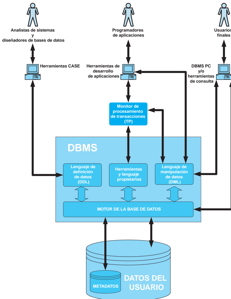
FIGURA 12.3 Arquitectura típica de un sistema de administración de base de datos
