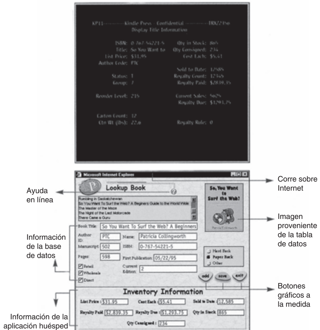
FIGURA 11.6 Diseño de una GUI a partir de una CUI
