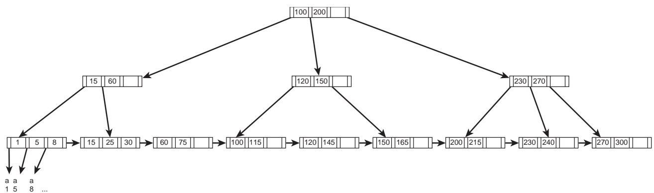
FIGURA A.14(b) Índice después de insertar 5 y borrar 80
