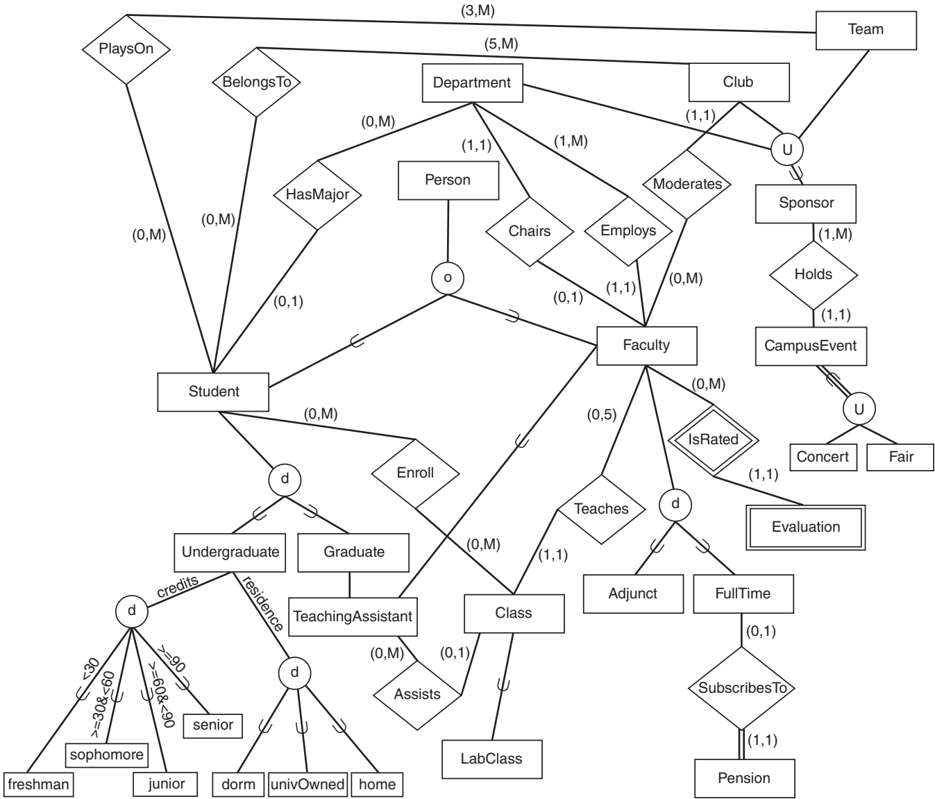
FIGURA 7.7 Diagrama EE-R para el ejemplo University
